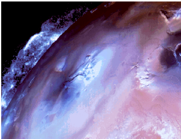
Извержения вулканов на Ио. Изображение с http://www.astronet.ru:8100/db/msg/1161681
