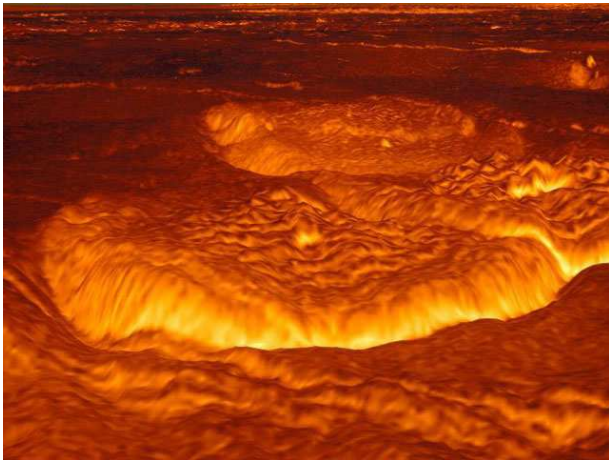
Горячая поверхность Венеры.
