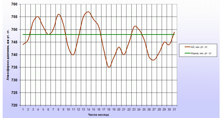
Прогноз хода атмосферного давления по г. Москве на январь 2009 г.
